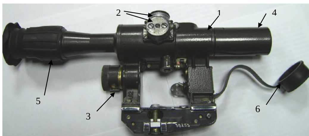
Рис. 102. Оптический прицел ПСО-1
