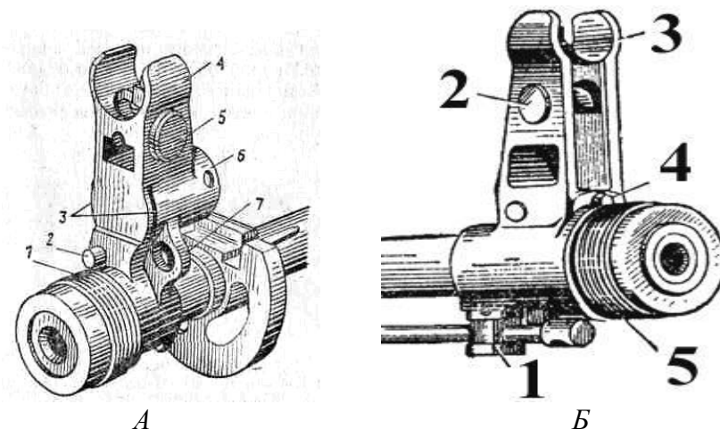
Рис. 12. Основание мушки: А – АКС-74У: 1 – резьба, 2 – фиксатор, 3 – пазы для установки накидной мушки приспособления для стрельбы ночью, 4 – предохранитель мушки, 5 – паз с мушкой; 6 – газовая камера, 7 – прилив с проушиной; Б – АК-74: 1 – упор для штыка-ножа, 2 – паз с мушкой, 3 – предохранитель мушки, 4 – фиксатор, 5 – резьба для навинчивания дульного тормоза-компенсатора
