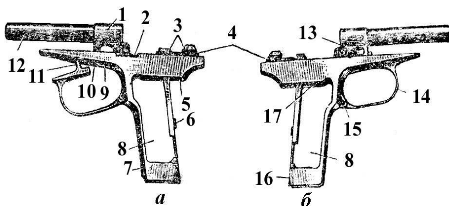
Рис. 29. Рамка со стволом и спусковой скобой:
