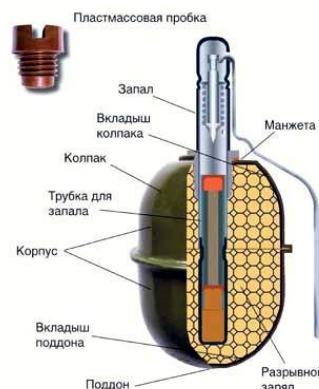
Рис. 71. Граната РГД-5
