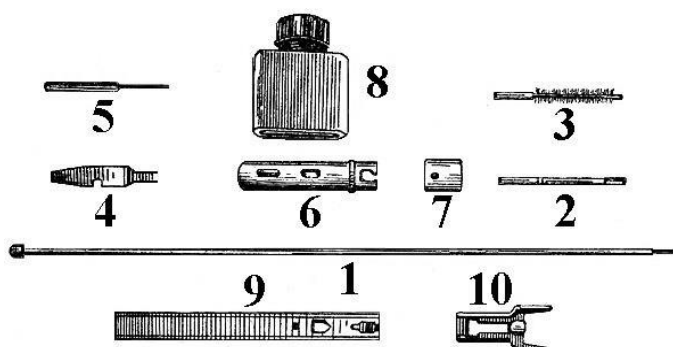
Рис. 10. Принадлежности к АК-74:
