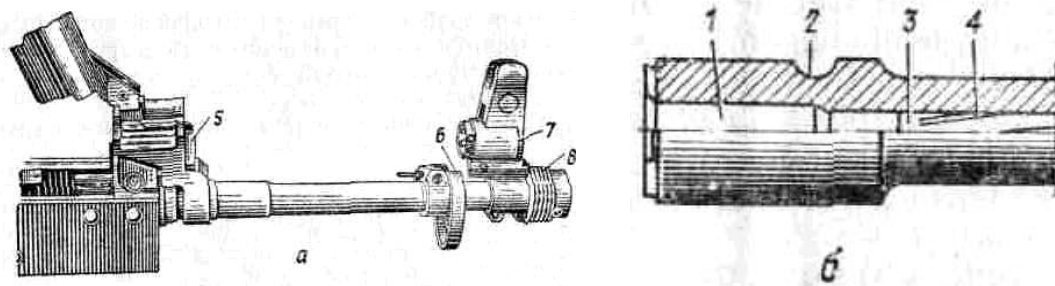
Рис. 14. Ствол:
