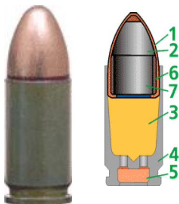
Рис. 56. Устройство патрона 9х19 мм «Парабеллум» («Люгер»): 1 – оболочка, 2 – пуля, 3 – пороховой заряд, 4 – гильза, 5 – капсюль, 6 – рубашка (обтюра- тор), 7 – стальной сердечник.
