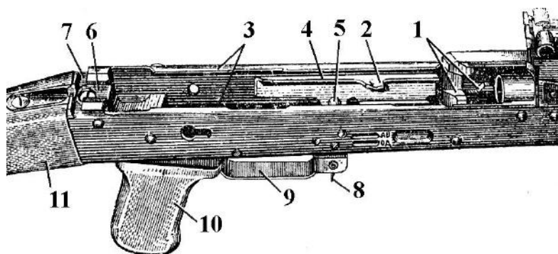
Рис. 16. Ствольная коробка:
