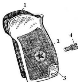
Рис. 41. Рукоятка с винтом:
