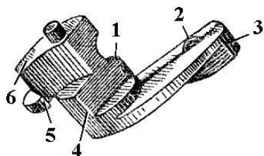
Рис. 33. Предохранитель: 1 – уступ, 2 – фиксатор, 3 – флажок, 6 – выступ предохранителя, 4 – ребро, 5 – зацеп
