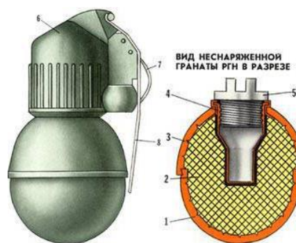
Рис. 72. Устройство РГН:
