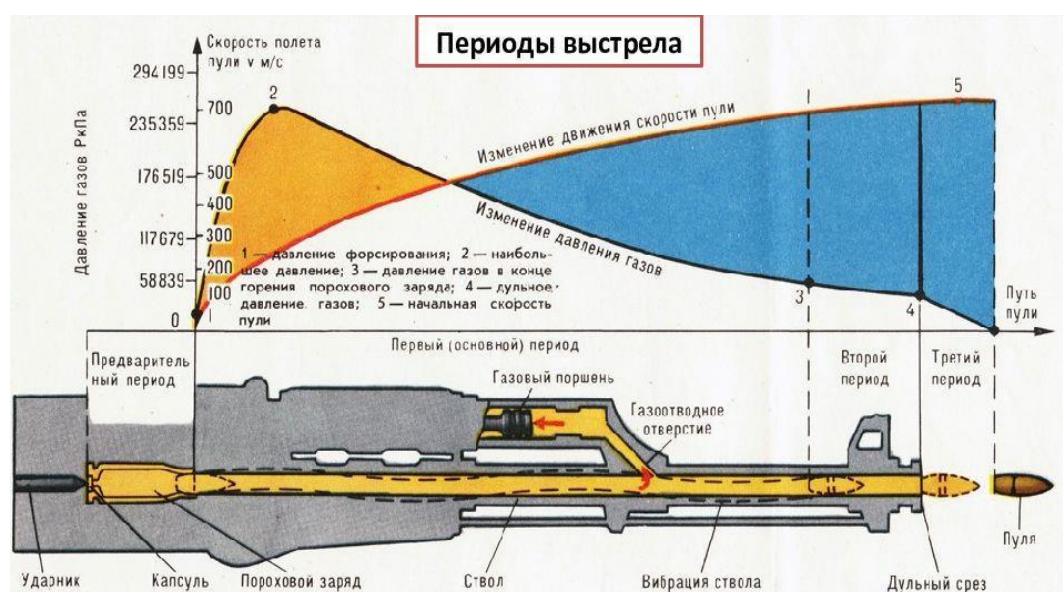
Рис. 1. Периоды выстрела
