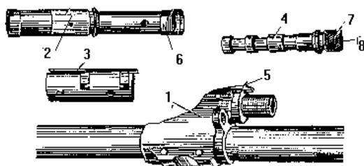
Рис. 60. Газовая камора:
