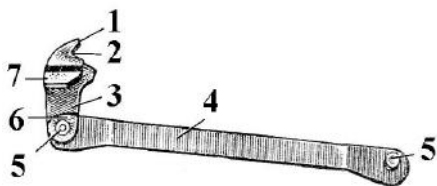
Рис. 36. Спусковая тяга с рычагом взвода: 1 – разобивающий выступ рычага взвода, 2 – вырез, 3 – рычаг взвода, 4 – спусковая тяга, 5 – цапфы спусковой тяги, 6 – пятачка рычага взвода, 7 – выступ самовзвода
