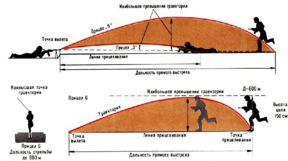
Рис. 3. Прямой выстрел
