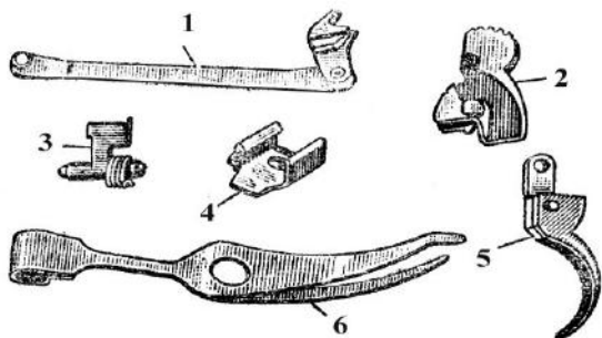
Рис. 35. Части ударно-спускового механизма:
