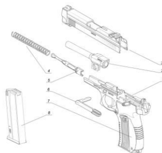
Рис. 47. Устройство пистолета Ярыгина
