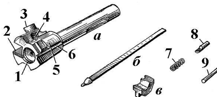
Рис. 18. Затвор:
