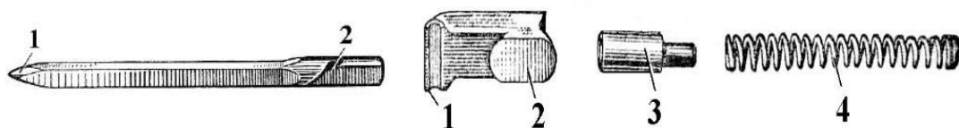
Рис. 31. Ударник: 1 – боек, 2 – срез для предохранителя
